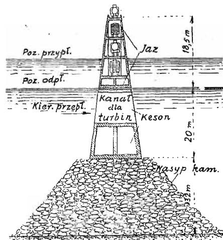
Rys. 3. Przekrój jazu.
